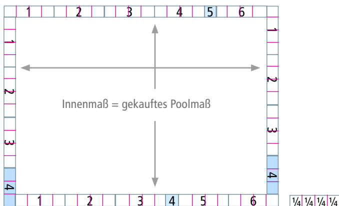
DRAUFSICHT Beispiel: Styroporpool 500 x 350 cm
